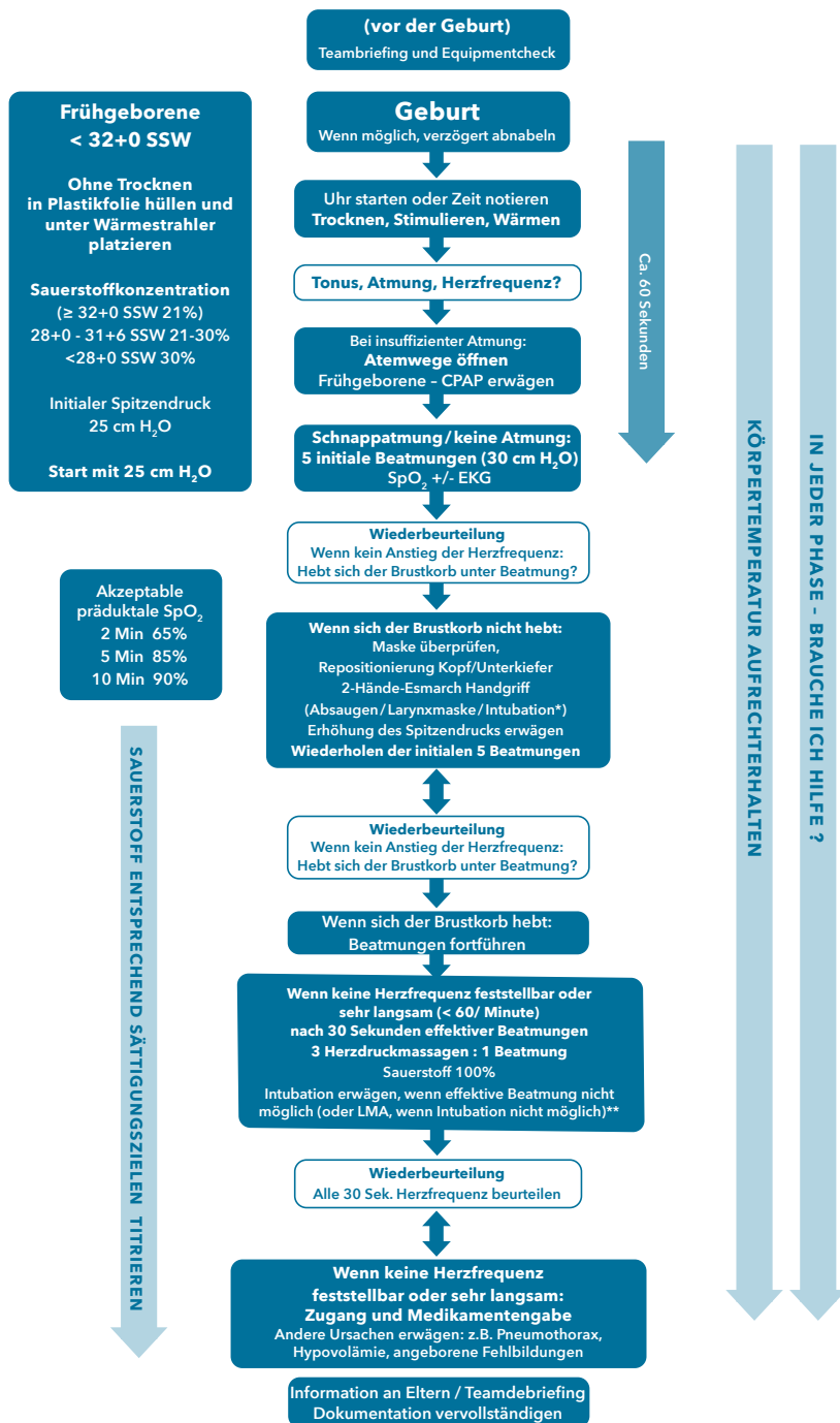
Abbildung 21 NLS-Algorithmus
