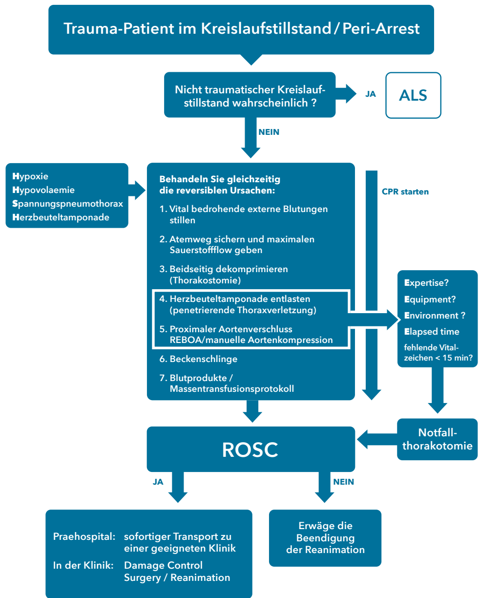
Abbildung 14 Trauma-Algorithmus
