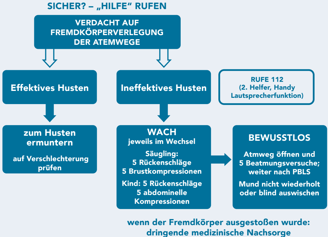
Abbildung 24 FBAO-Algorithmus
